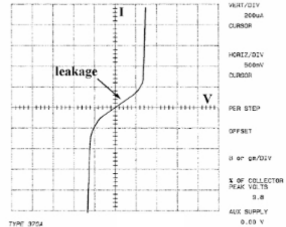
洩漏
