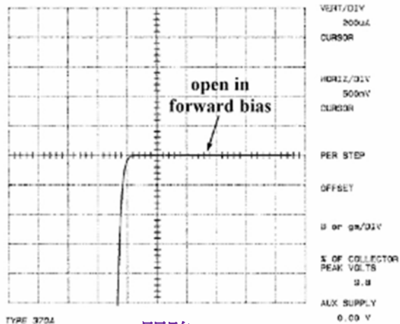
開路
