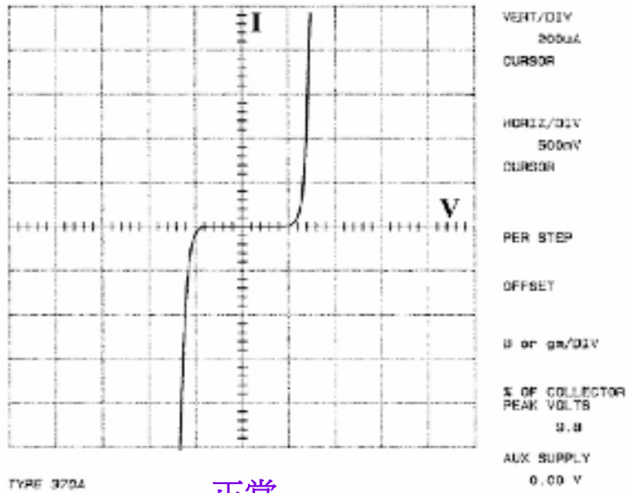
正常
